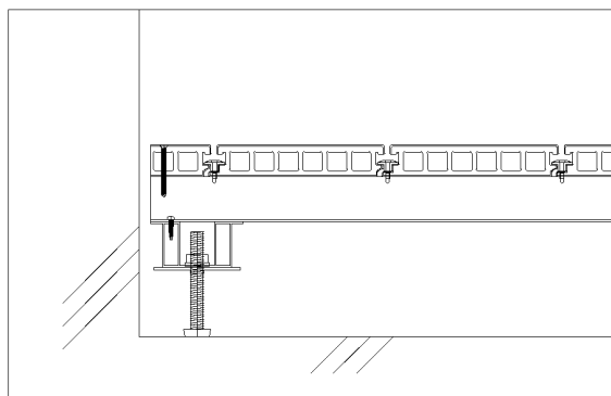
図2 緩衝材付ボルト
